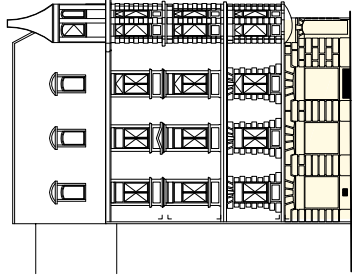
Ansicht Bodmerstrasse
