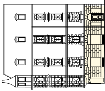
Ansicht Alfred-Escher-Strasse
