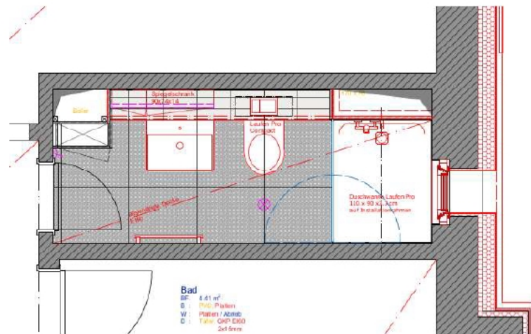
Bad Rechts 1. - 3. OG Grundriss
