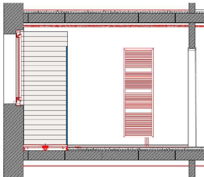
Bad Rechts 1. - 3. OG Ansicht B
