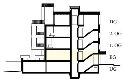
Schnitt
