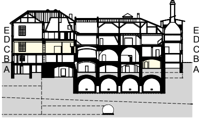
Schnitt
