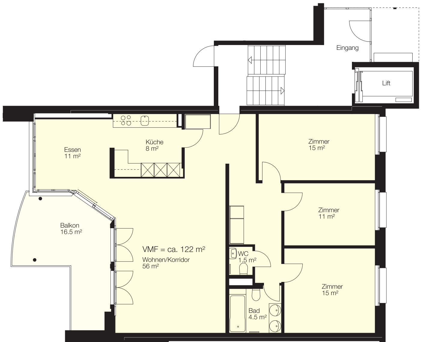
Grundriss
