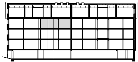
Schnitt
