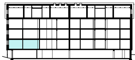
Schnitt
