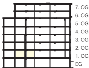
Schnitt
