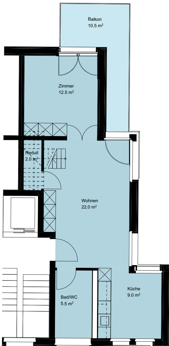
Grundriss
