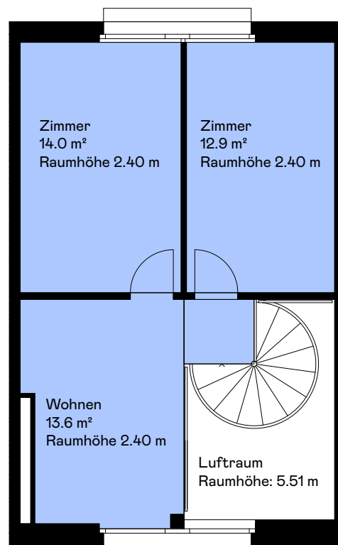
Galeriegeschoss
