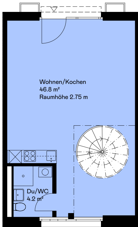
Eingangsgeschoss
